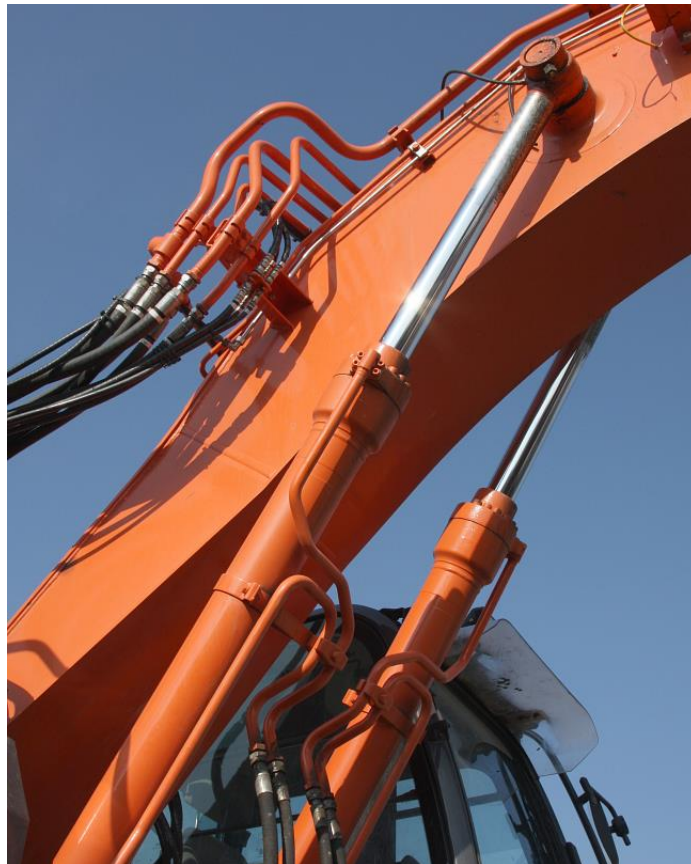
Bild1: Hydraulikzylinder im Einsatz an einem Bagger (Holger Müller)
